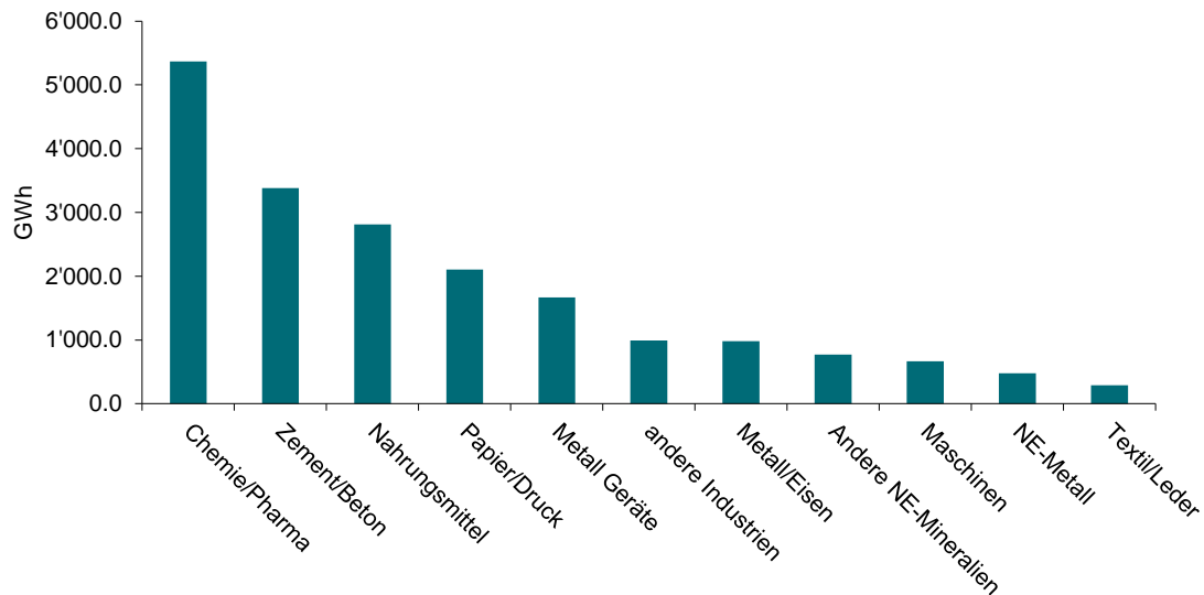
Figur 7: Jährlicher Verbrauch von thermischer Energie pro Branche 2012 (Bachmann 2013)
