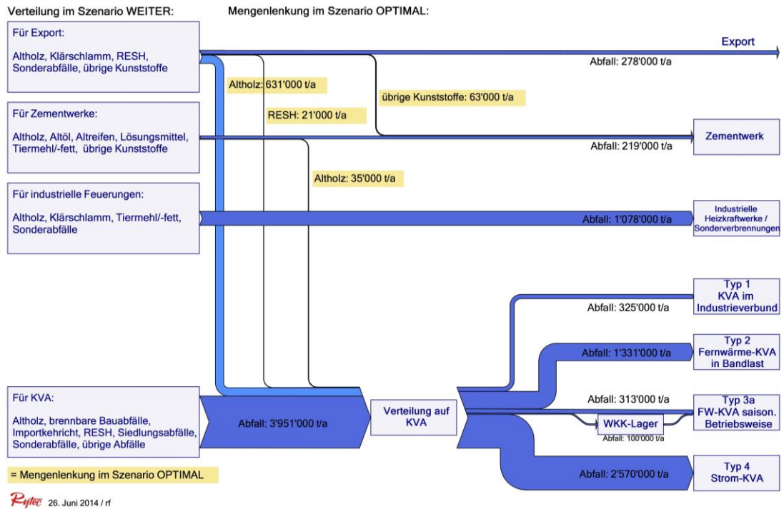
Figur 17: Resultat der Lenkung der relevanten Stoffströme auf die Verwertungsanlagen im Szenario «optimierte Abfallwirtschaft» 2035. Gelb hinterlegt die «aktiv gelenkten» Stoffströme.
