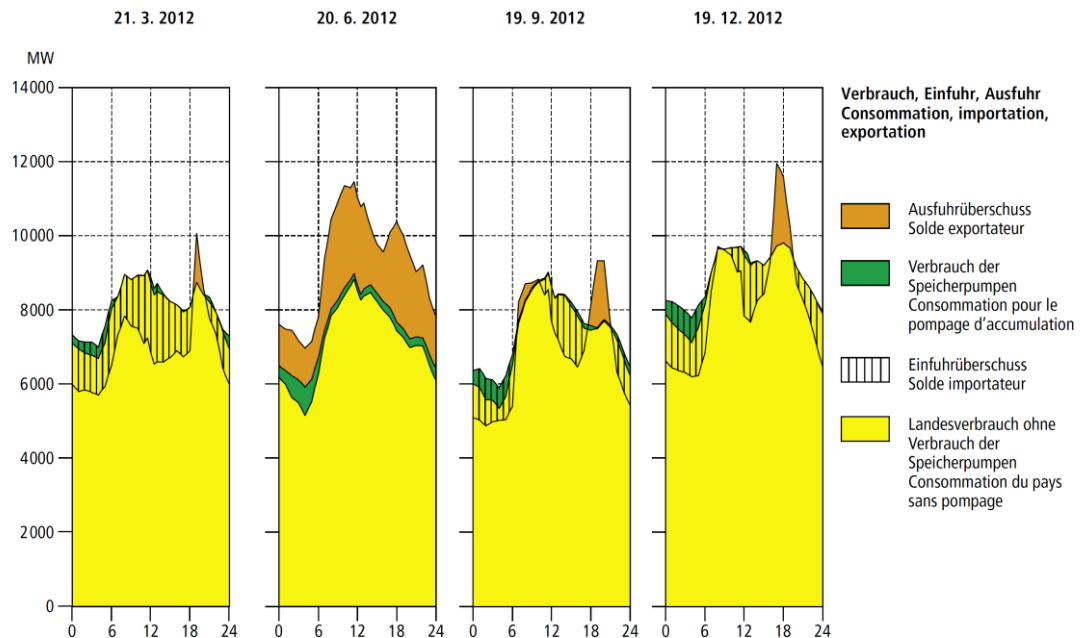
Figur 11: Belastungsverlauf am dritten Mittwoch des Monats (BFE 2013a)
