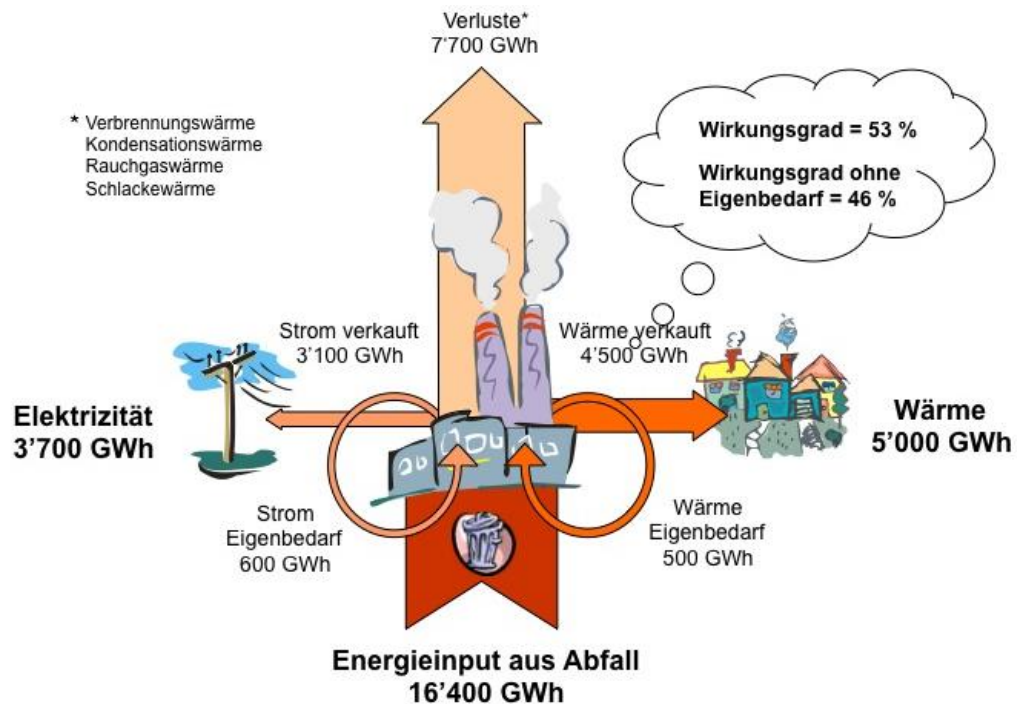
Figur 21: Auswirkungen der Stoffstromlenkung im Szenario «optimierte Abfallwirtschaft» auf den Energiefluss der Schweizer KVA im Jahr 2035.
