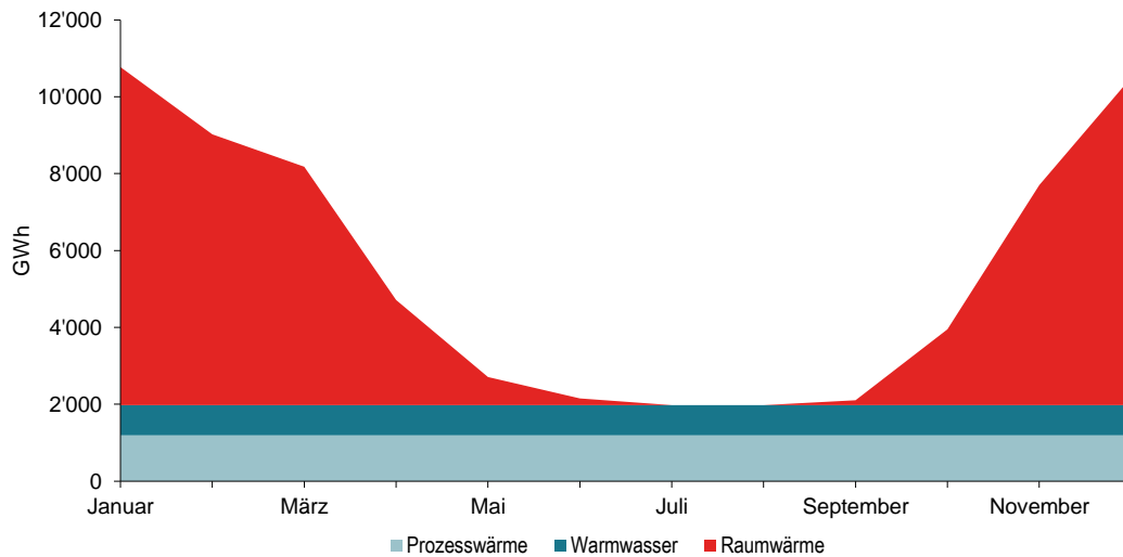
Figur 8: Szenario «Neue Energiepolitik»: Wärmeverbrauch (Raumwärme/Warmwasser/Prozesswärme, ohne elektrische Produktion) in GWh pro Monat 2035
