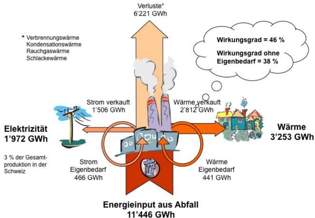
Figur 5: Illustrative Darstellung der Energieströme durch Schweizer KVA im Jahr 2012. Durch Optimierungsmassnahmen wird der Gesamtwirkungsgrad laufend gesteigert. Der Wirkungsgrad (ohne Eigenbedarf) beträgt heute bei der Elektrizität 13% und der Wärme 25%.
