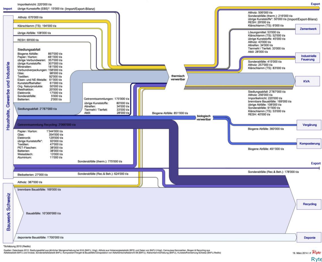
Figur 1: Darstellung der Massenströme in der Schweizer Abfallwirtschaft in Tonnen pro Jahr. Werte 2012. Die Anhänge 4 und 5 zeigen sämtliche Sankey-Diagramme in vergrößerter Darstellung.
