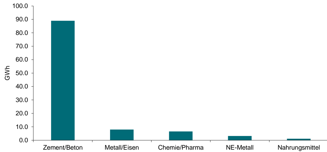
Figur 27: Durchschnittlicher Verbrauch von thermischer Energie pro Betrieb in ausgewählten energieintensiven Branchen 2012 (Bachmann 2013)
