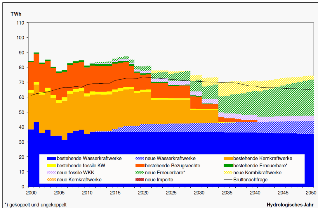
Figur 12: Szenario «Neue Energiepolitik», Variante C&E*: Perspektiven der Elektrizitätsversorgung, hydrologisches Jahr (TWh el ) (Prognos 2012a)
