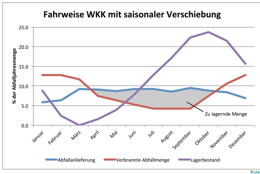
Figur 28: Abfallanlieferung im Jahrgang und Abfallverbrennung die dem Fernwärmebedarf nachgefahren wird mit resultierendem Lagerbestand.
