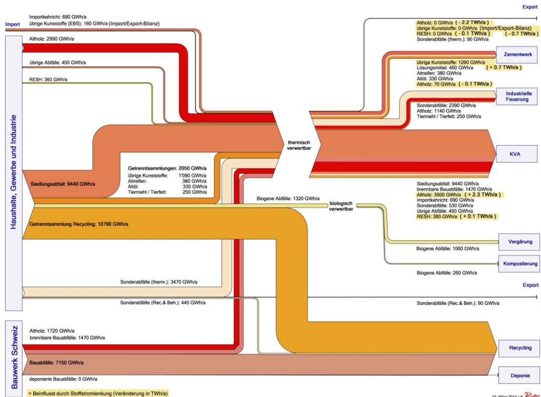
Figur 19: Energieflüsse in der optimierten Abfallwirtschaft 2035 in GWh pro Jahr (Eine vergrösserte Version befindet sich in Anhang A-5)
