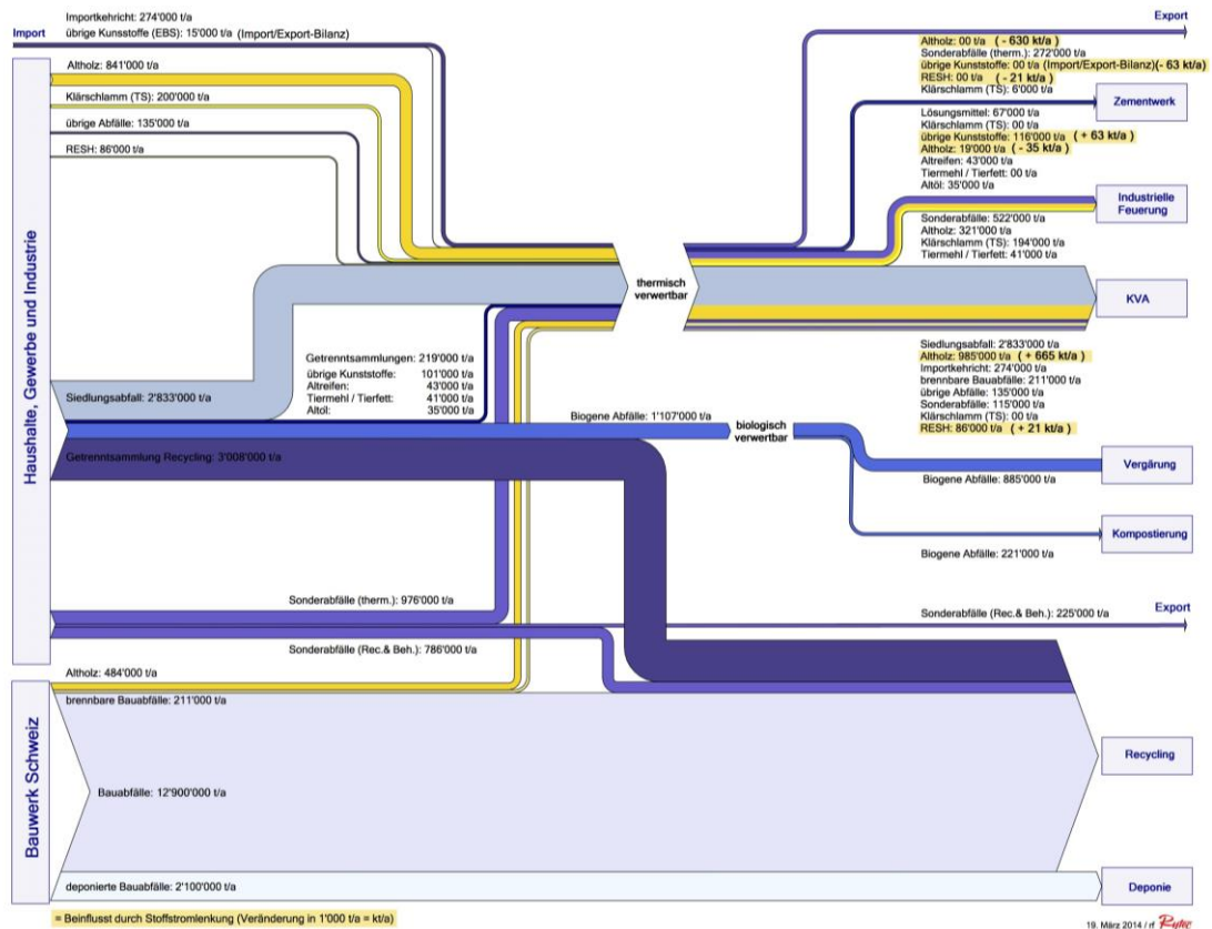
Figur 18: Massenflüsse in der optimierten Abfallwirtschaft 2035 in Tonnen pro Jahr (Eine vergrößerte Version befindet sich in Anhang A-4)
