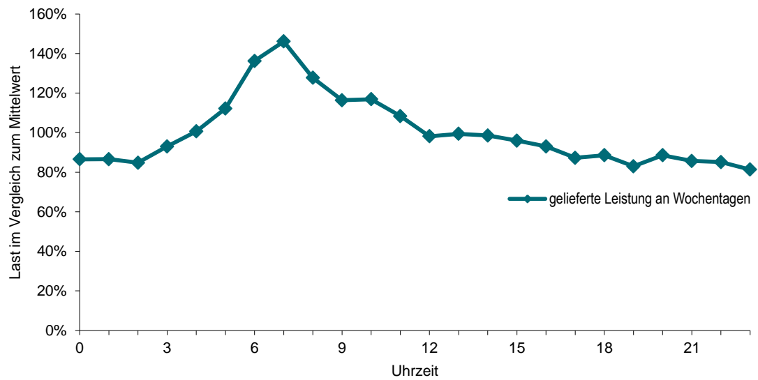
Figur 26: Typischer Tagesverlauf der gelieferten Leistung in % des Mittelwertes einer Fernwärmeversorgung ab KVA
