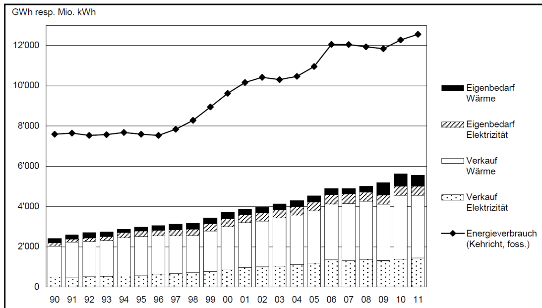
Thermische Stromproduktion in der Schweiz
