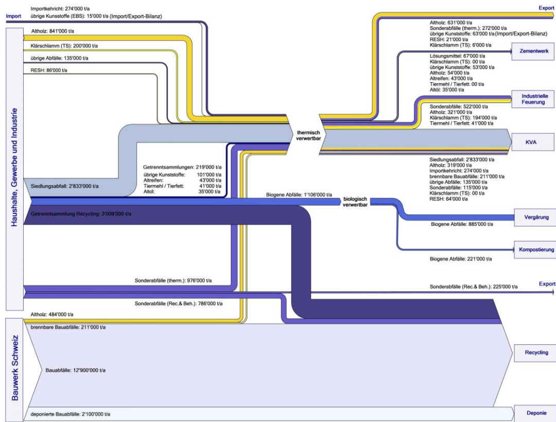
Figur 15: Darstellung der Massenströme in der Schweizer Abfallwirtschaft in Tonnen pro Jahr. Ungelenkte Entwicklung «Weiter wie bisher». Eine vergrößerte Darstellung befindet sich im Anhang A-4.
