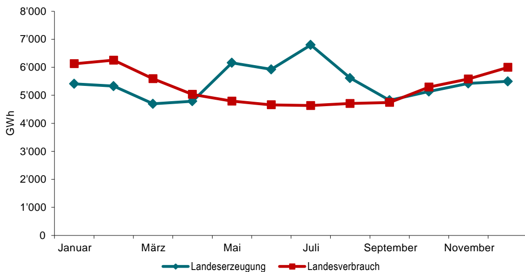
Figur 10: Gesamte Erzeugung (abzüglich Verbrauch der Speicherpumpen) und Verbrauch (inkl. Verluste) elektrischer Energie in der Schweiz (2012) (BFE 2013b)
