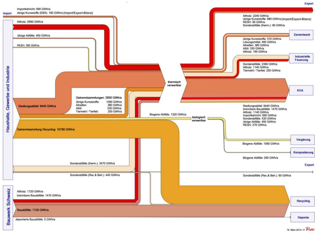
Figur 16: Darstellung der Energieströme in der Schweizer Abfallwirtschaft in GWh pro Jahr. Ungelenkte Entwicklung «Weiter wie bisher». Eine vergrösserte Darstellung befindet sich im Anhang A-5.
