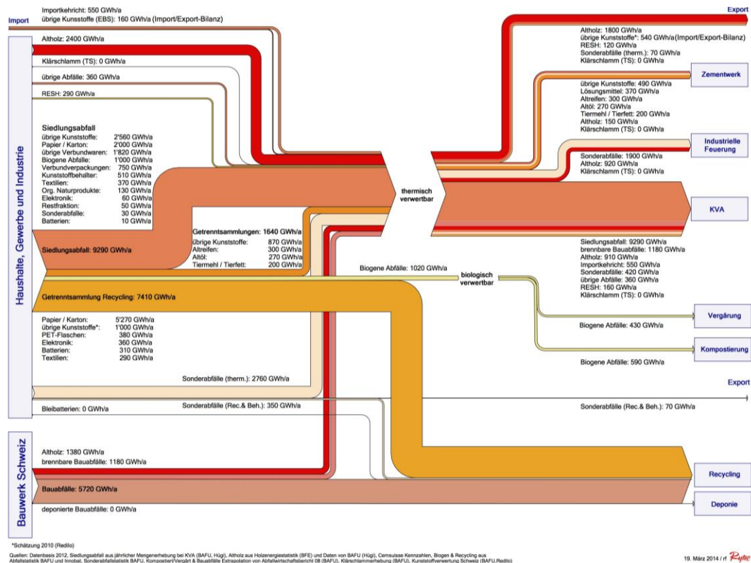
Figur 3: Energieflüsse in GWh pro Jahr, die für eine optimierte Energienutzung betrachtet werden können (Stand 2012). Eine vergrösserte Darstellung befindet sich im Anhang A-5.
