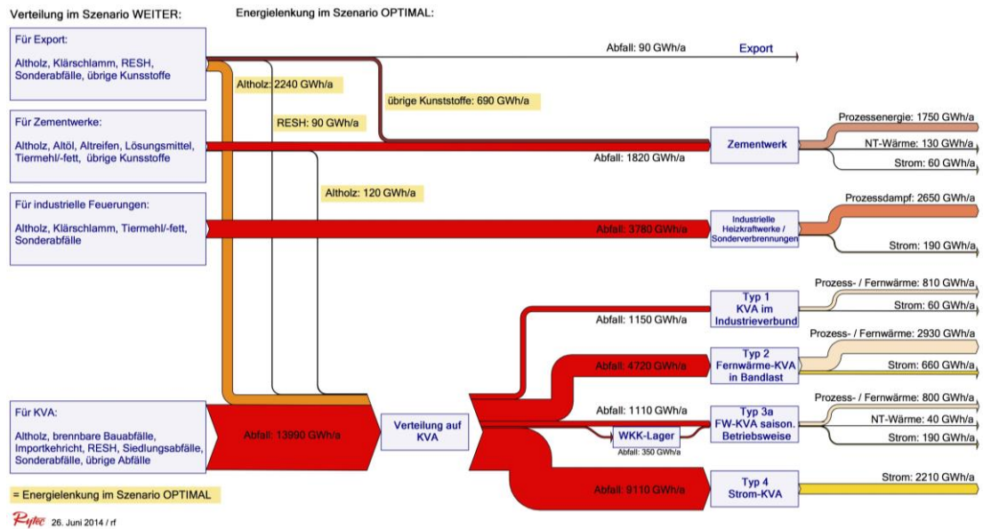
Figur 20: Zuordnung der Energieflüsse auf die Anlagentypen in der optimierten Abfallwirtschaft 2035 (siehe Anhang A-14 für die Gesamtdaten)
